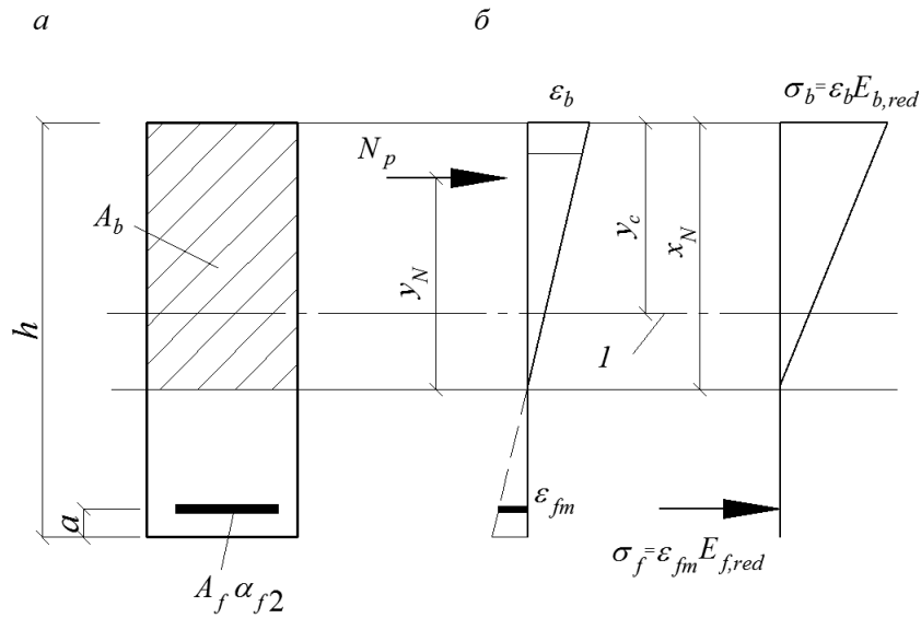
1 — уровень центра тяжести приведенного без учета растянутой зоны бетона поперечного сечения
