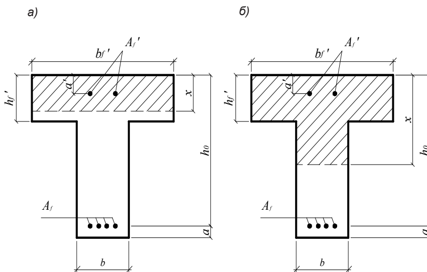
Рисунок 2 — Положение границы сжатой зоны в сечении изгибаемой конструкции
