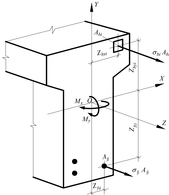
Рисунок 5 — Расчетная схема нормального сечения конструкции
