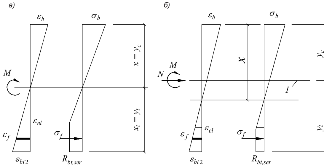
1 — Уровень центра тяжести приведенного поперечного сечения
